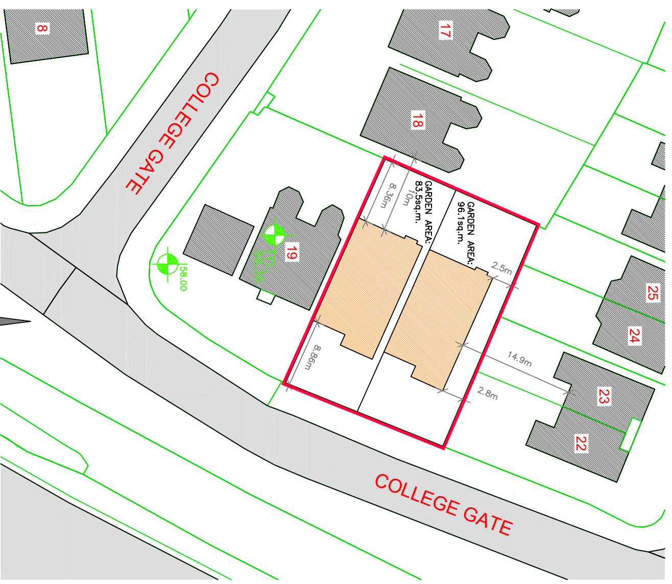
SITE MAP 1:500
