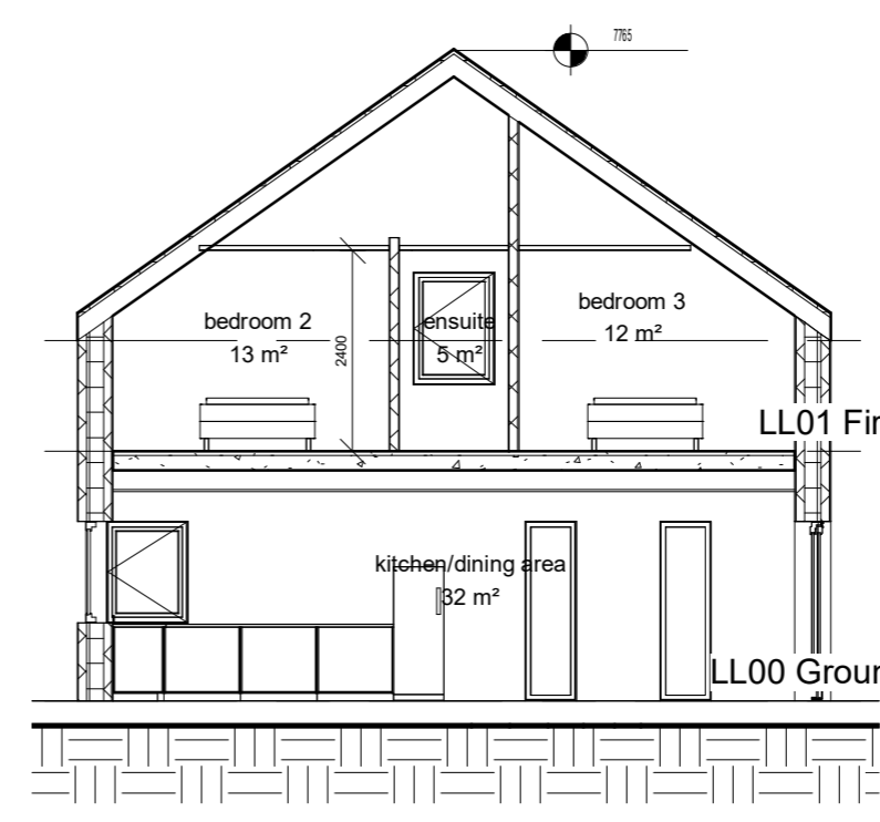
2 Section 1 1 : 100
